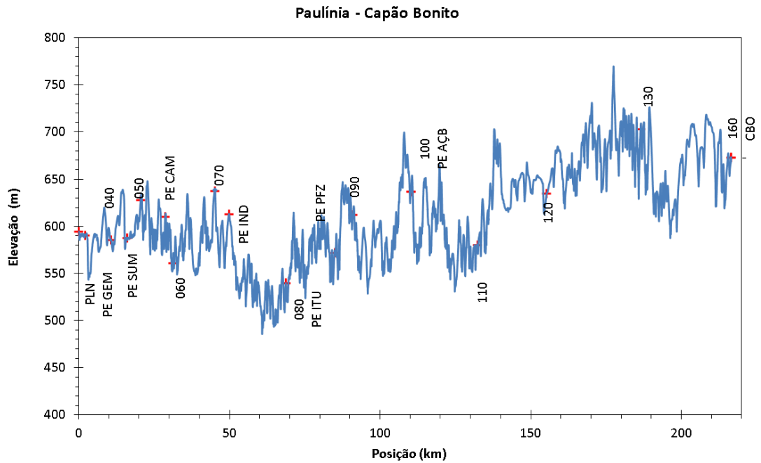
Figura 8 – Perfil altimétrico do trecho Paulínia-Capão Bonito
