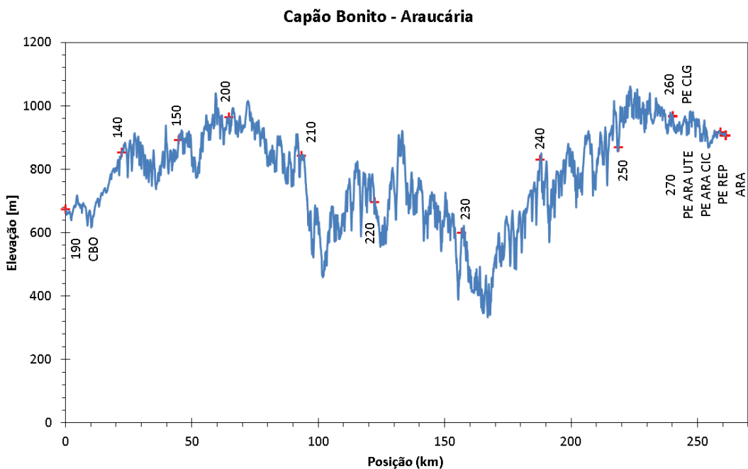
Figura 9 – Perfil altimétrico do trecho Capão Bonito-Araucária
